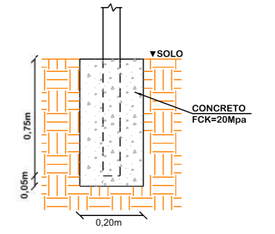
DETALHE DE FIXAÇÃO AO SOLO PARA PLACAS DE REGULAMENTAÇÃO E ADVERTÊNCIA 0,80x0,20x0,20m
