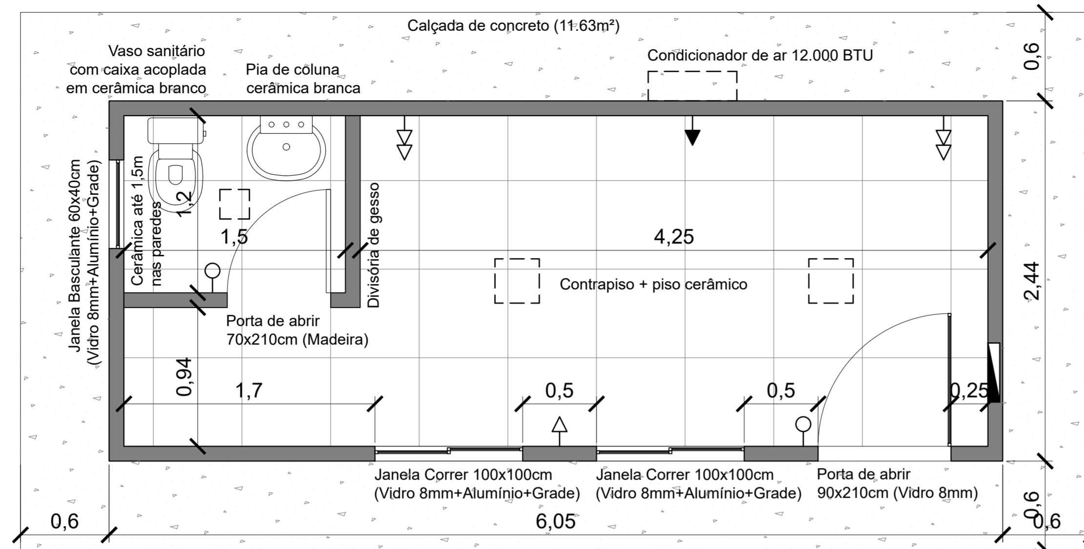
PLANTA BAIXA Escala 1/25
