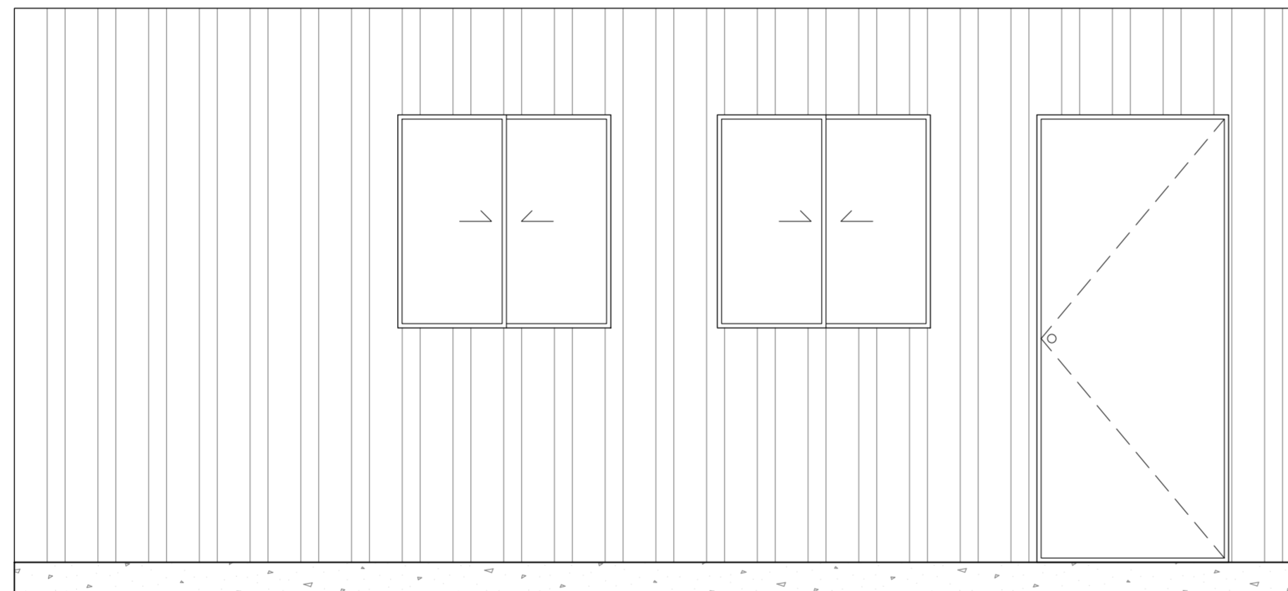
ELEVAÇÃO FRONTAL Escala 1/25
