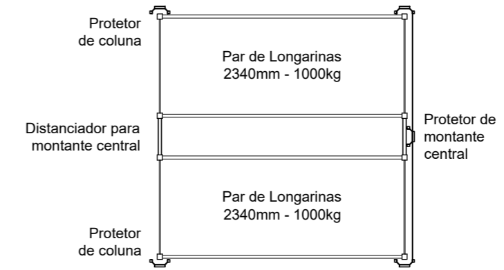
VISTA SUPERIOR DE FILEIRA DUPLA Escala 1/50
