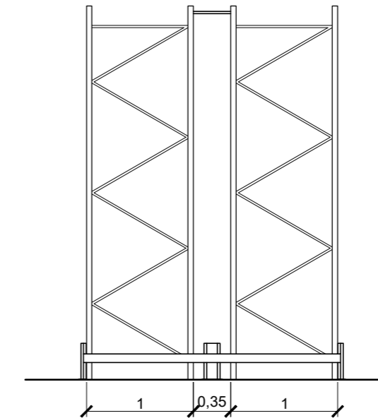
VISTA LATERAL DE FILEIRA DUPLA Escala 1/50
