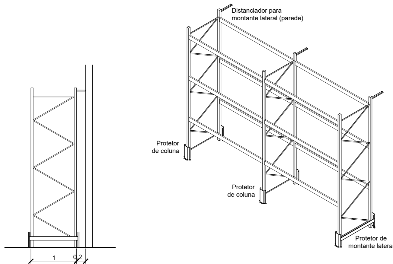
VISTA LATERAL DE FILEIRA DE PAREDE Escala 1/50
