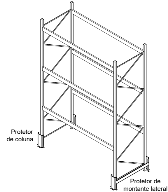
PERSPECTIVA ISOMÉTRICA DE UM MÓDULO Escala 1/50
