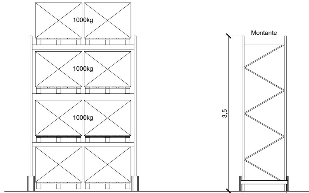
VISTA FRONTAL DE UM MÓDULO Escala 1/50
