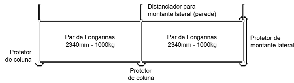
VISTA SUPERIOR DE FILEIRA DE PAREDE Escala 1/50
