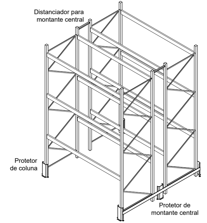
PERSPECTIVA ISOMÉTRICA DE FILEIRA DUPLA Escala 1/50
